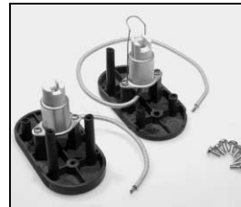
L4.77152.E Lamp holder set Lampenfassung
