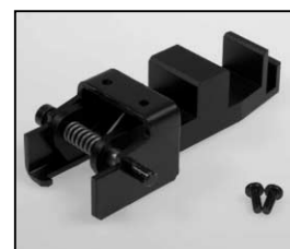
L4.82038.E Top latch "long version" Torsicherung "lange version"
