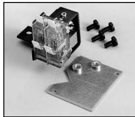
L4.77539.E Safety switch complete Endschalter komplett
