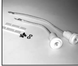
L4.72586.E H.T. cables cpl. thread: 20mm from ser.no.1609 Lampenkel kpl. Gewinde: 20mm ab Ser.Nr. 1609
