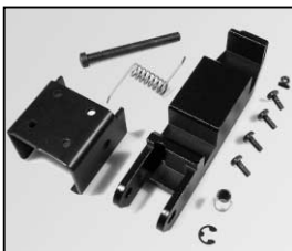
L4.77470.E Top latch "middle" (in combination with accessory brackets L4.77344.E) Torsicherung "mittel" (in Verbindung mit Halteklauen L4.77344.E)
