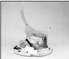
L4.75801.E to / bis ser. no. 117 Thread / Gewinde: 17 mm Spindle / Spindel Ø 12 Lamp holder + lamp carriage Lampenfassung + Fokusschlitten
