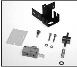
L4.77399.E Safety switch complete Endschalter komplett
