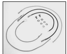
L4.86255.E Connecting wires Ballast/Ignitor Verbindungslitzen Vorschalt gerät/Zündgerät
