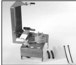
L4.86525.E Lampholder + lamp carriage Lampenfassung + Fokusschlitten
