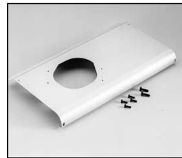
L4.82202.E to/bis Ser.No.1981 Side panel right 200–240 V Seitenblech rechts 200–240 V
