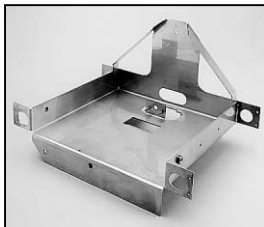
L4.82289.E Lamp carriage Fokusschlitten
