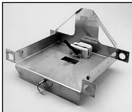
L4.82279.E Lampholder + lamp carriage Lampenfassung + Fokusschlitten
