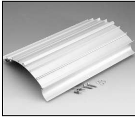
L4.82477.E Extrusion right to ser. no. 250 Rippenblech rechts bis Ser. Nr. 250
