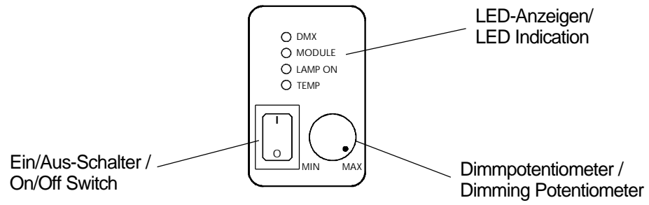
Abb./Fig. 4: Bedienelemente 200 W-Modul/ Operating Parts 200 W-Module
