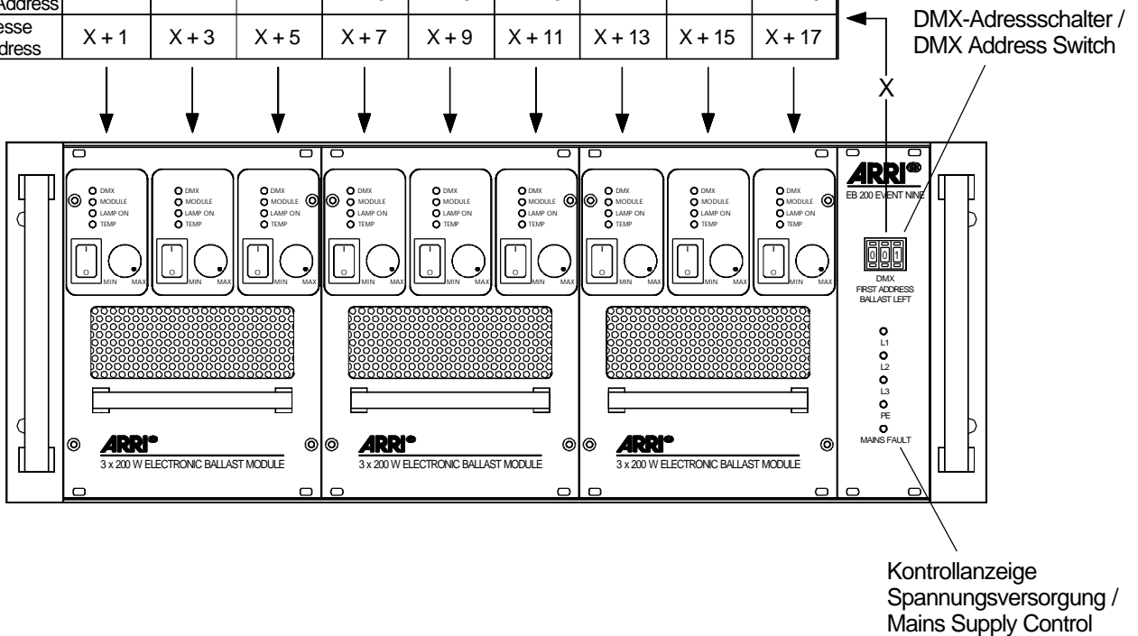
Abb./Fig. 3: Ansicht Gerätefront / Front View of Ballast
