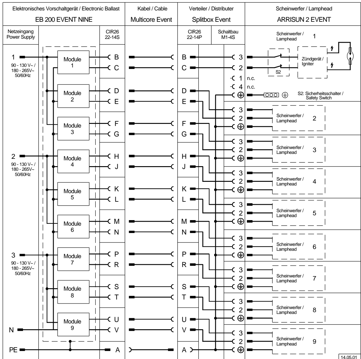
Abb./Fig. 1: Elektronisches Vorschaltgerät mit Scheinwerfern / Electronic Ballast with Lamp Units
